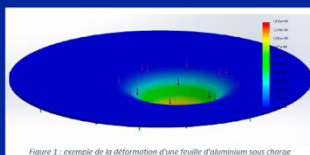
Figure 1 : exemple de la déformation d'une feuille d'aluminium sous charge
